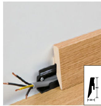
Fußleiste Profil 3 PK (60 mm)
