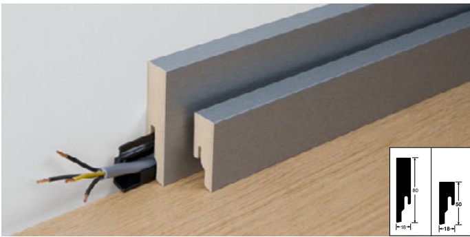
Fußleiste Profil 9 PK (80 mm), Profil 8 PK (50 mm)
