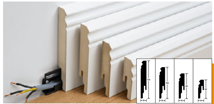
Fußleiste Profil 13 PK (120 mm), 12 PK (100 mm), 11 PK (80 mm), 10 PK (60 mm)
