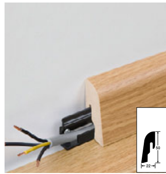
Fußleiste Profil 2 PK (50 mm)
